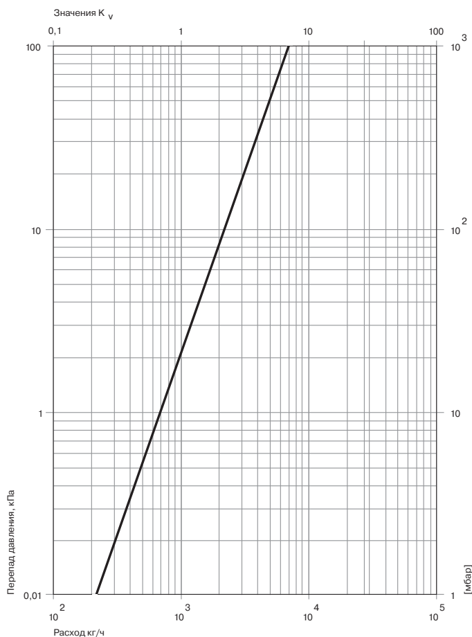
Для однотрубной системы отопления
