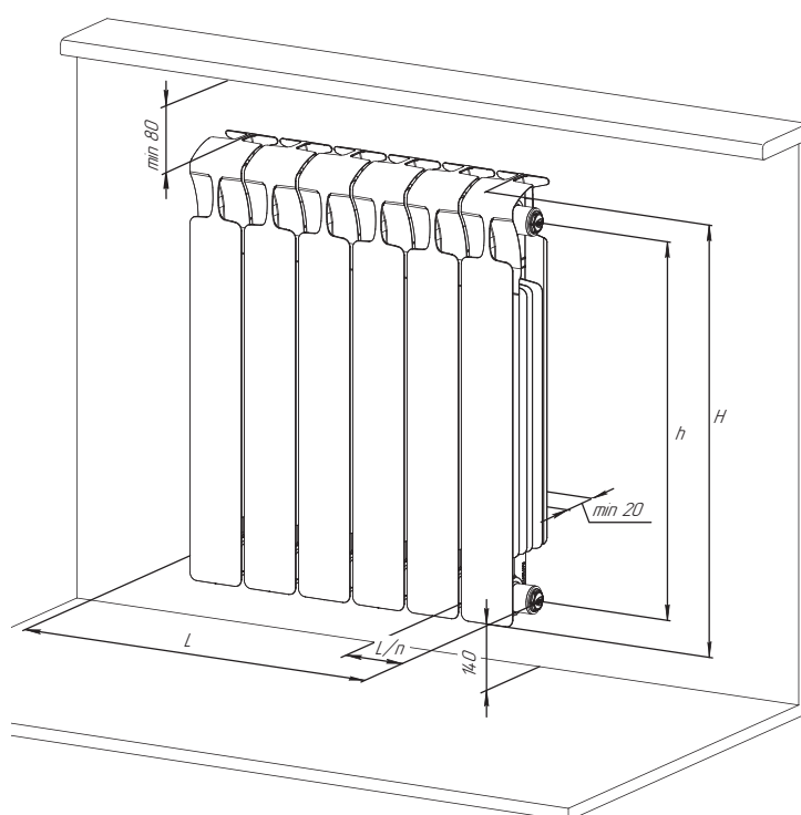
Рис 1. Схема настенного монтажа радиатора
